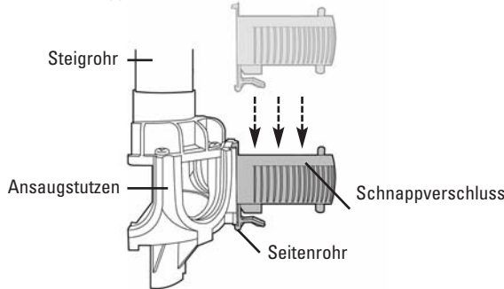
ABBILDUNG 1 - Schnappverschluss-Detail
