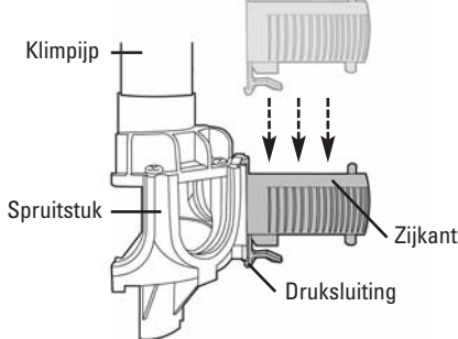
AFBEELDING 1 drukvast detail.
