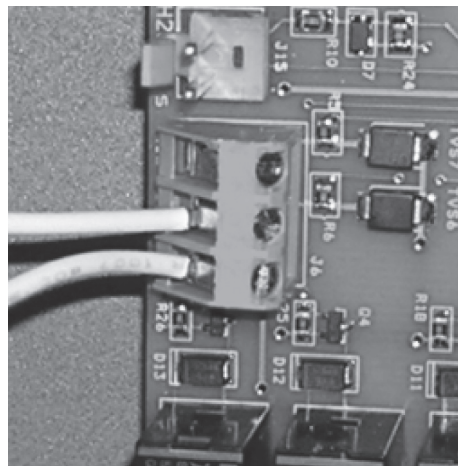
Figure 11b. Connexion à AquaLink® RS ou TSTAT à distance (Connexion à 2 fils)
