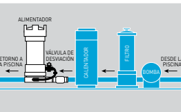
Ilustración del clorinador de tabletas modelo 320
